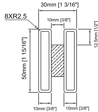
A-A Detail
